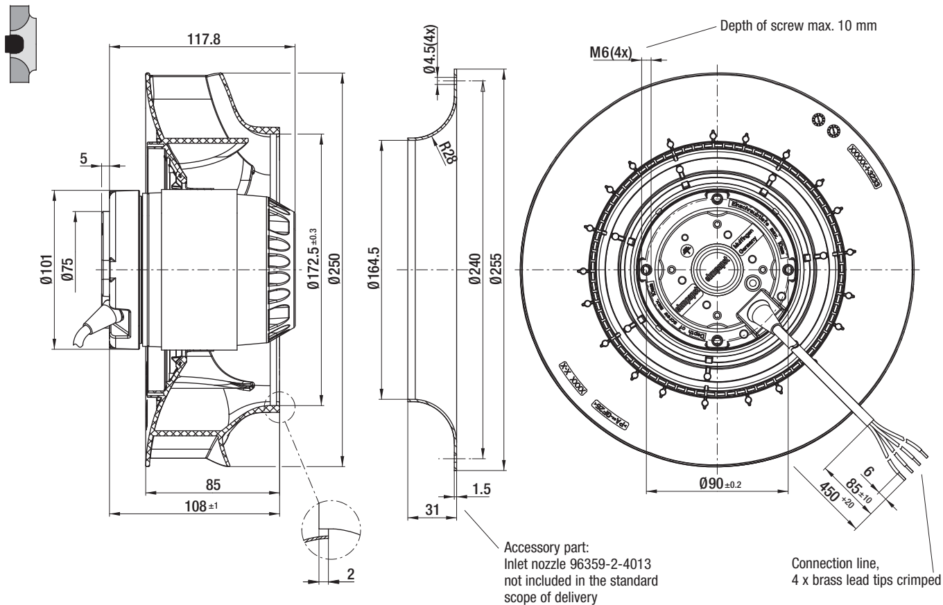
R2E 250-RB06-01 (Centrifugal fan)
